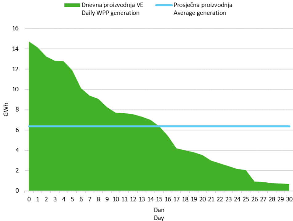
Slika 6 Krivulja trajanja dnevne proizvodnje vjetroelektrana u ožujku 2021. godine
