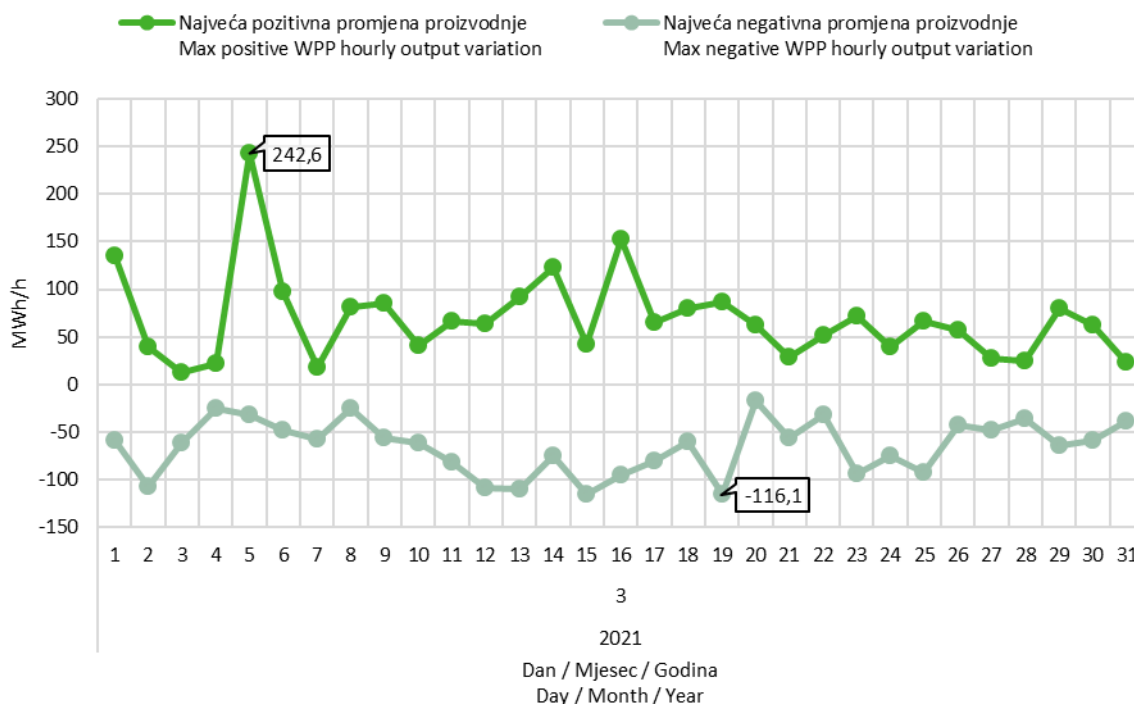
Slika 9 Maksimalna pozitivna i maksimalna negativna promjena satne proizvodnje VE u ožujku 2021. godine
