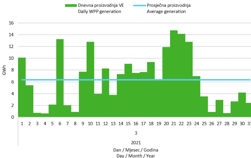
Slika 5 Dnevna proizvodnja svih vjetroelektrana u ožujku 2021. godine
