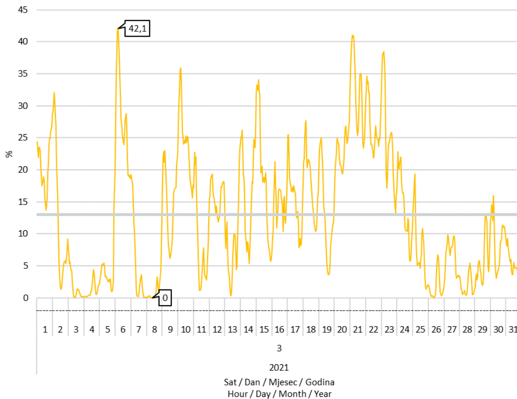
Slika 8 Udio proizvodnje vjetroelektrana u pokrivanju satnog opterećenja elektroenergetskog sustava u ožujku 2021. godine
