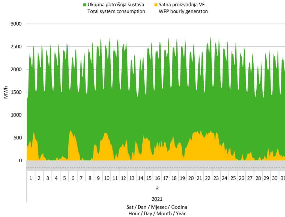
Slika 7 Usporedba satnog dijagrama opterećenja sustava i proizvodnje vjetroelektrana u ožujku 2021. godine
