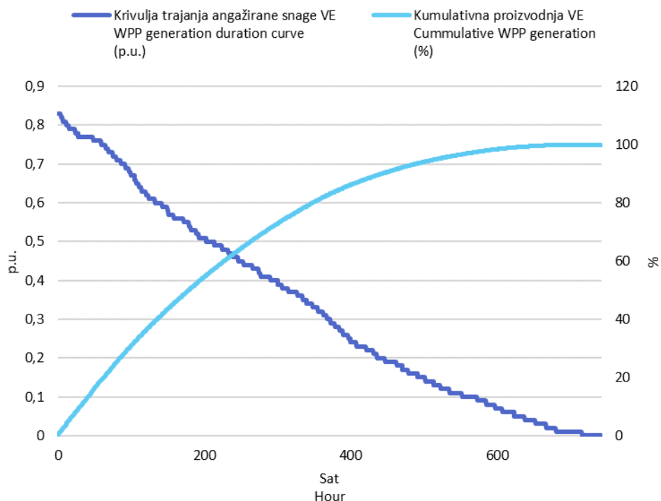
Slika 3 Krivulja trajanja angažirane snage svih VE i kumulativna proizvodnja VE u ožujku 2021. godine u jediničnim vrijednostima
