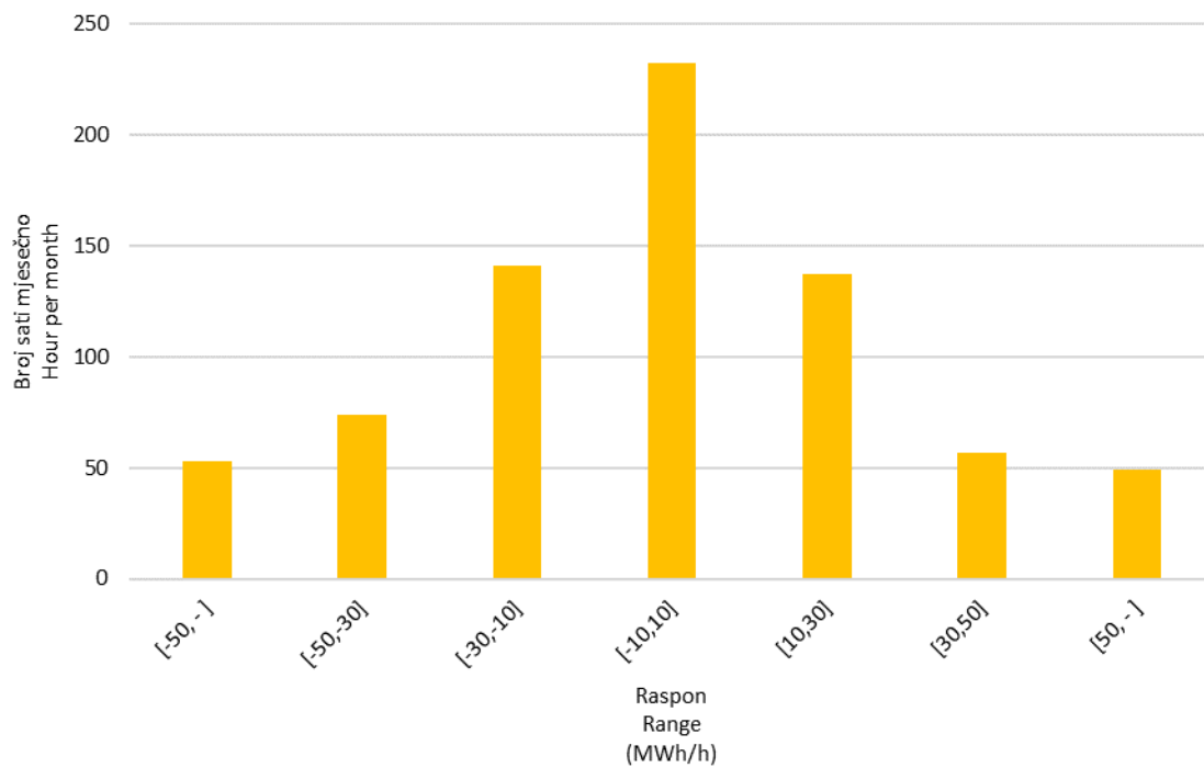
Slika 10 Statistička raspodjela satnih promjena proizvodnje VE u ožujku 2021. godine
