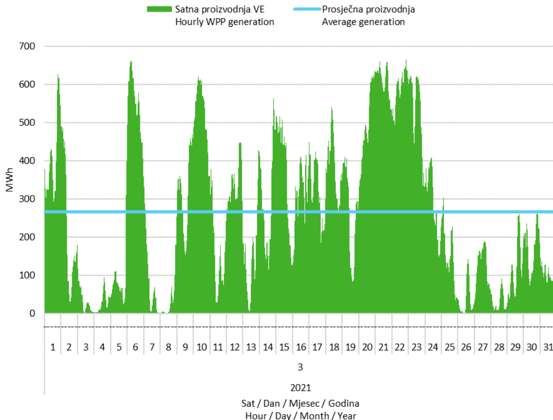
Slika 2 Satna proizvodnja svih vjetroelektrana u ožujku 2021. godine
